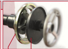
GAR 122 GAR 114 (Ø 202-221-281) Completa di coni per autocarri Complete with cones for trucks Komplett mit Spannzubehör für LKW Équipée de cônes PL. Completa de conos para camiones
