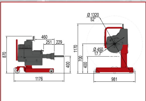
GAR 122 GAR 114 (Ø 202-221-281) Completa di coni per autocarri Complete with cones for trucks Komplett mit Spannzubehör für LKW Équipée de cônes PL. Completa de conos para camiones
